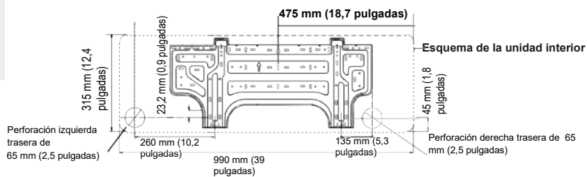
Modelo C Esquema de la unidad interior
