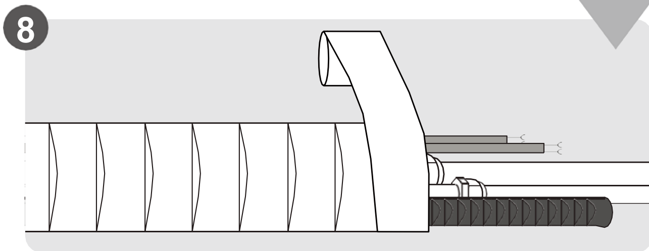
Envolver la tubería y los cables (Página 18)
