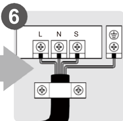
Conectar los cables (Página 17)
